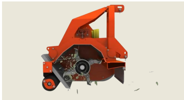
Rake kit . Ρυθμιζόμενες κόντρα λεπίδες υπό γωνία
